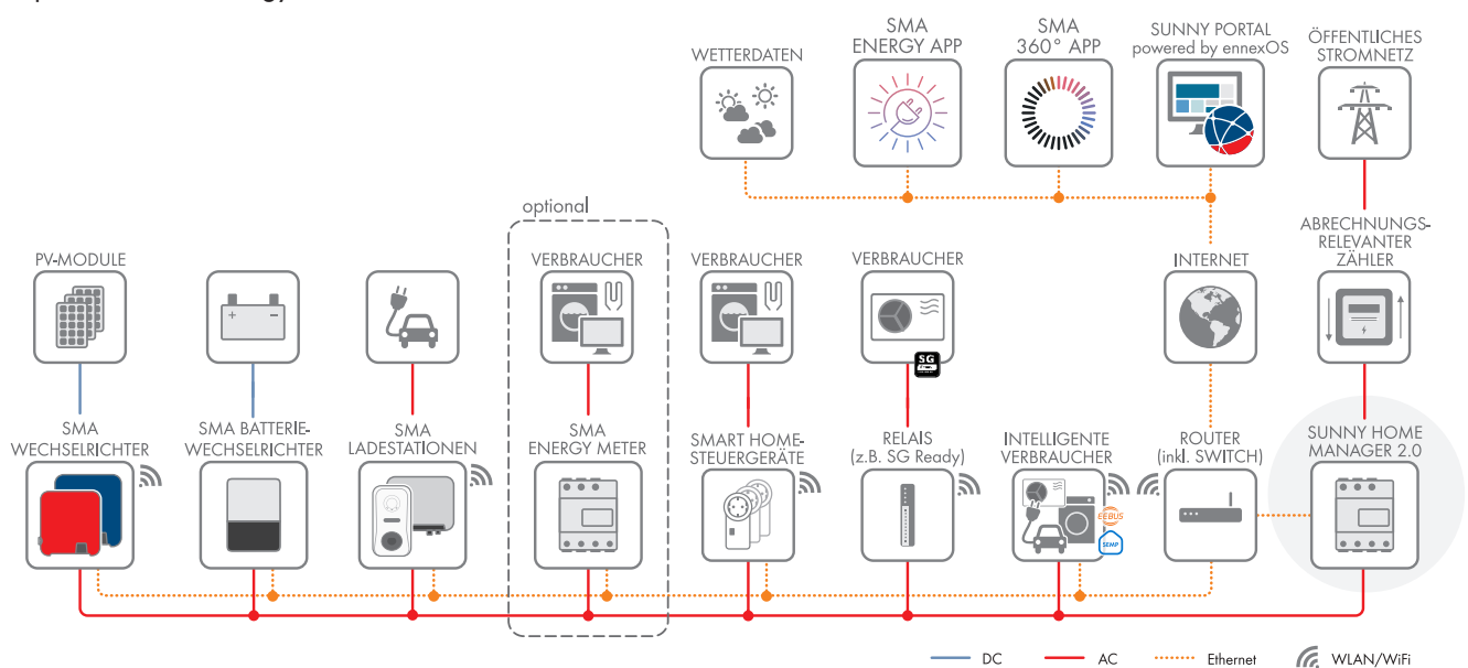
Abbildung 4: Betrieb der PV-Anlage mit SMA Wechselrichtern
